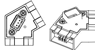
CONECTOR 120° ALIMENTACIÓN
