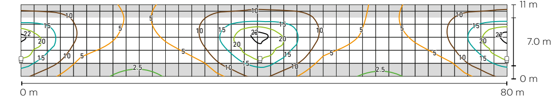
ARREGLO DE 3 LUMINARIAS
